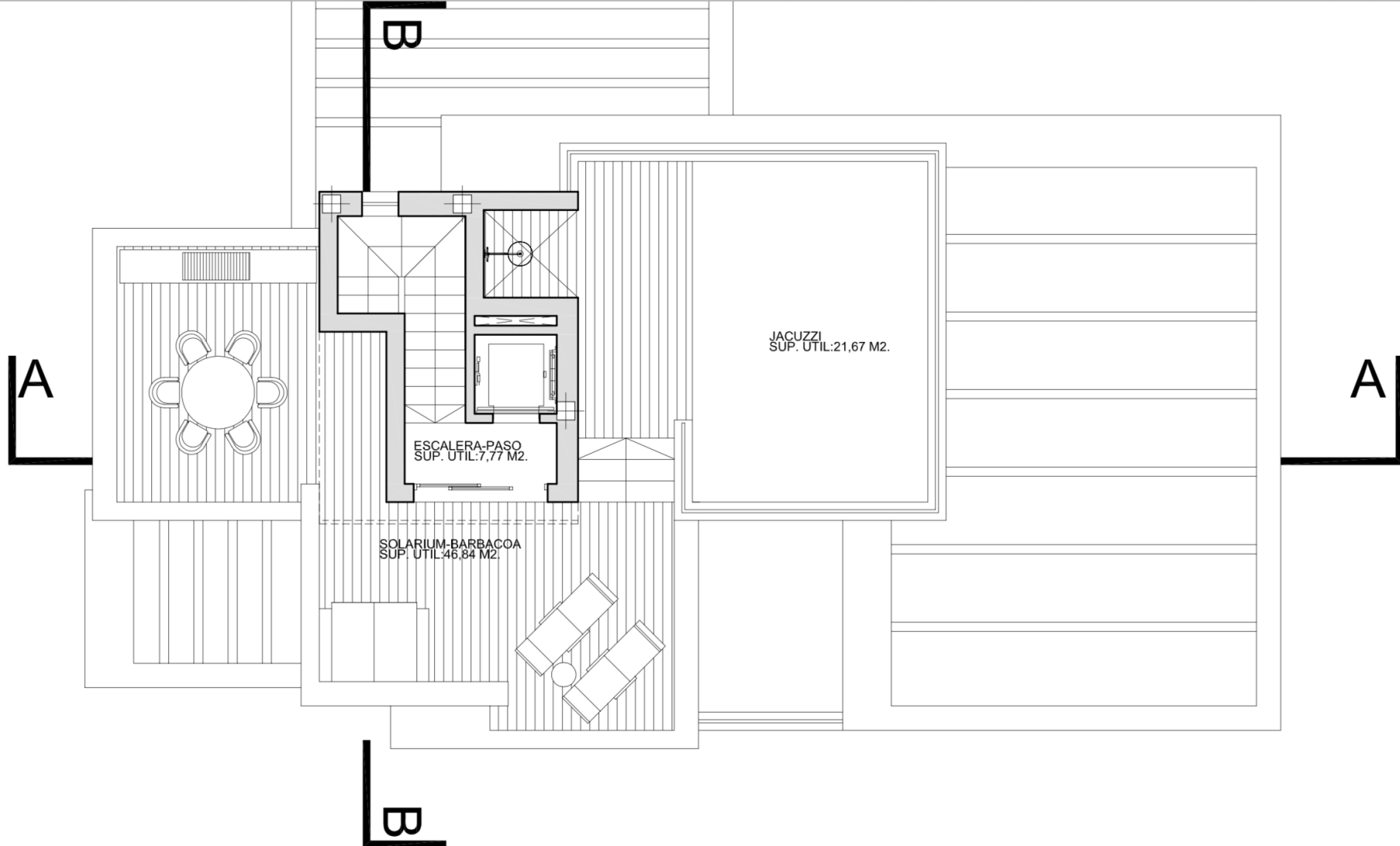
PLANTA SOLARIUM
